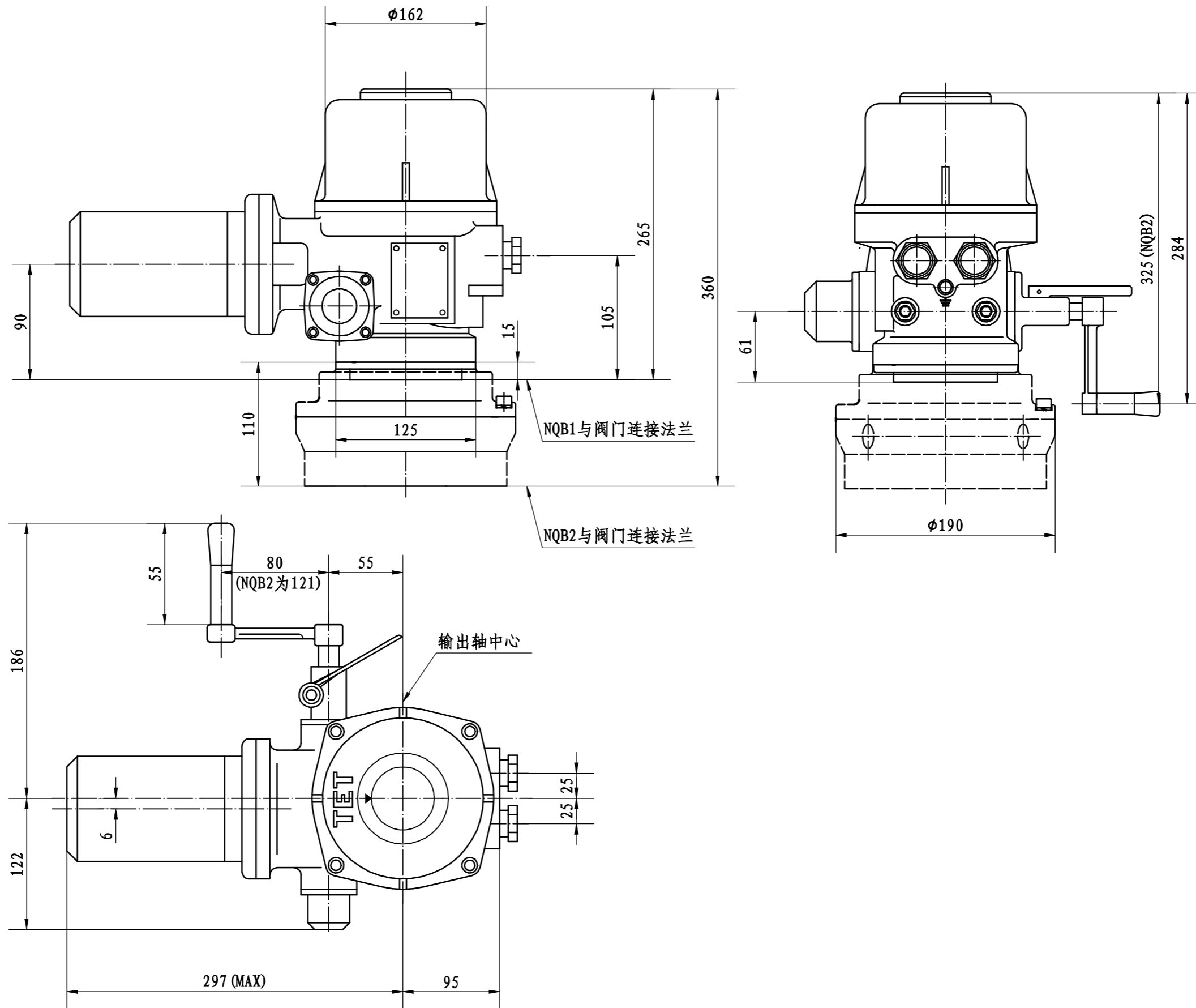
NQB1、NQB2普通型产品外形尺寸图
